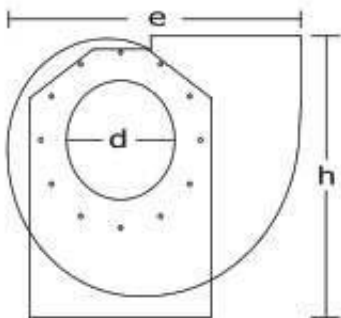
Ø250-1.5HP-1450RPM
